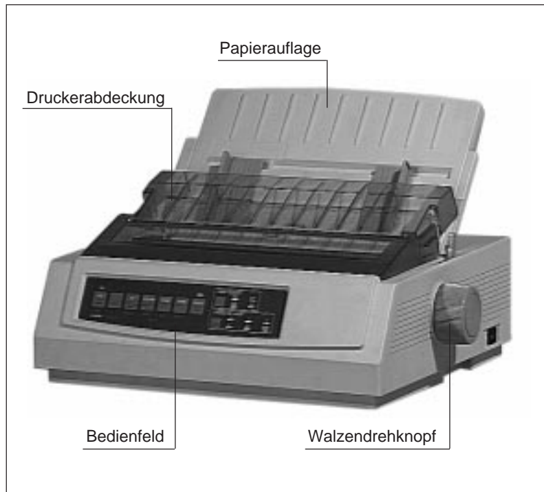
Vorderansicht
