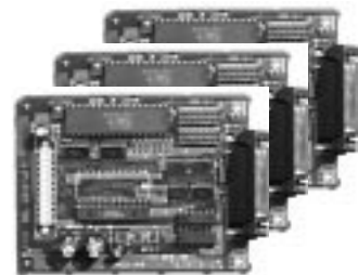
Serielle Schnittstellen: RS-232C, RS-232C / Current Loop, RS-422A
