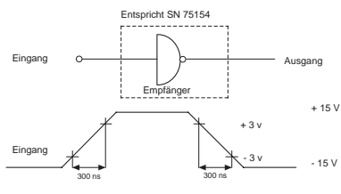
Eingangsschaltung
